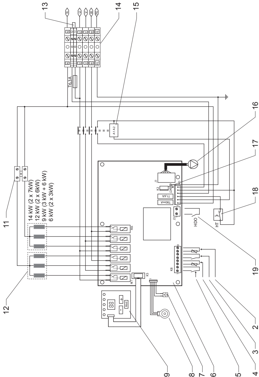
Электрическая схема котла ПРОТHERM Скaт 14 (12, 9, 6) кВт
